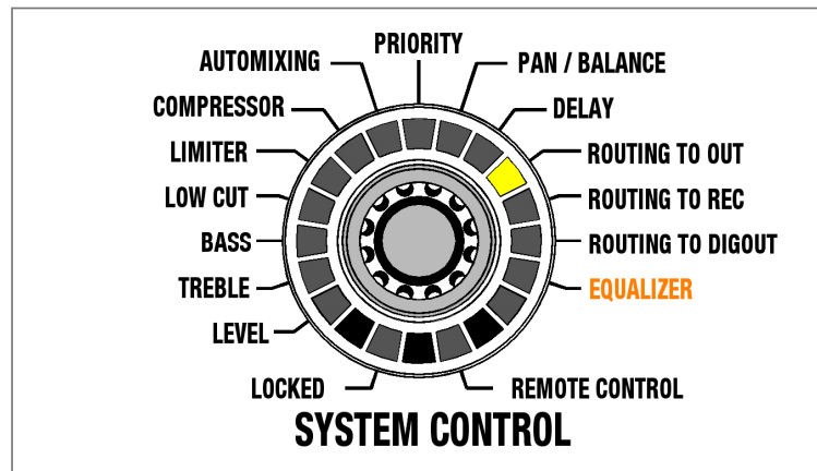
Abbildung 49: ROUTING TO OUT Funktion
