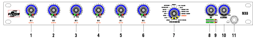
Abbildung 1: Frontseite des MX6
