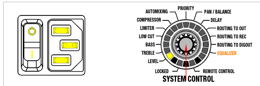
Abbildung 59: Rücksetzen auf Werkseinstellungen
