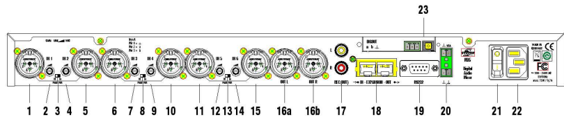
Abbildung 2: Rückseite des MX6
