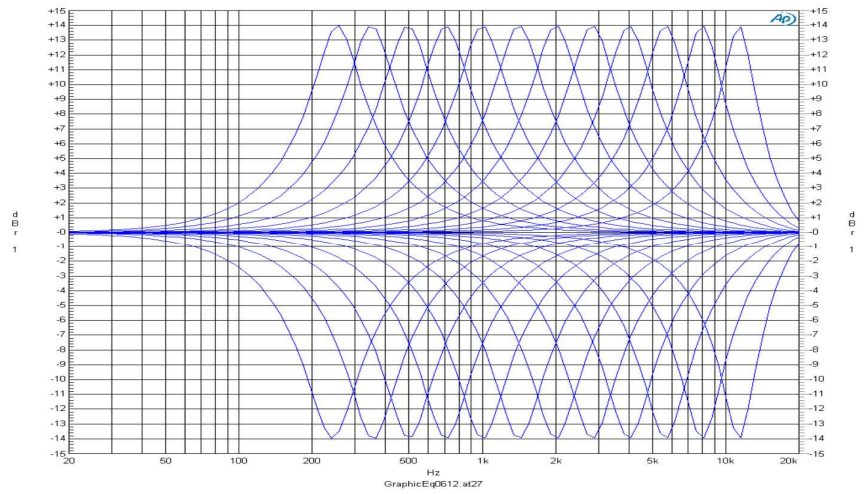
Abbildung 58: Regelmöglichkeit der EQUALIZER Funktion
